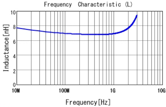
■ LQG15WH6N8J02 L
