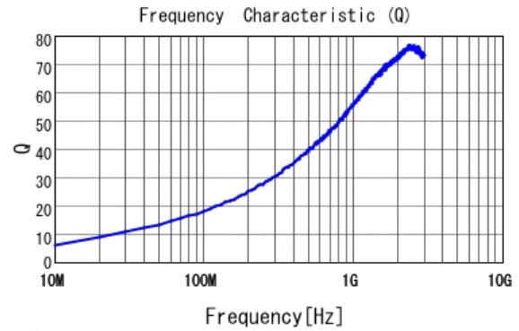
■ LQG15WH5N6B02 Q
