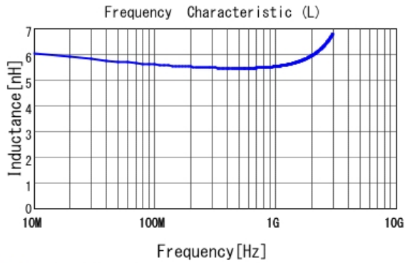
■ LQG15WH5N6B02 L
