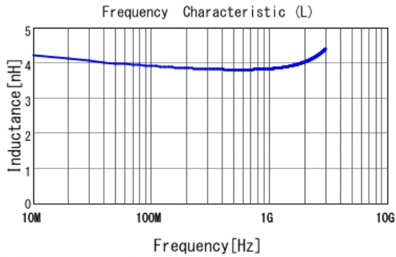
■ LQG15WH3N9B02 L
