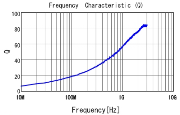
■ LQG15WH3N9B02 Q
