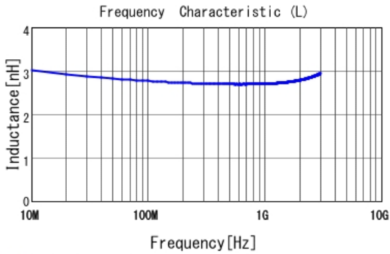
■ LQG15WH2N7B02 L
