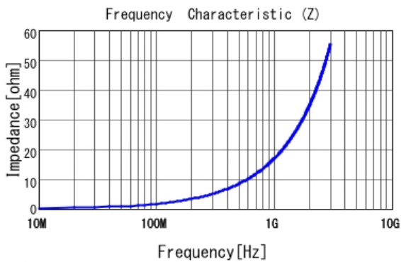
■ LQG15WH2N7B02 |Z|
