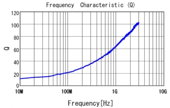
■ LQG15WH2N7B02 Q
