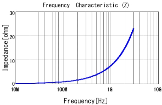
■ LQG15WH1N2B02 |Z|
