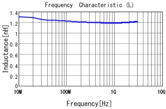
■ LQG15WH1N2B02 L
