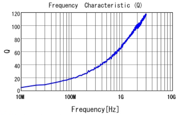
■ LQG15WH1N2B02 Q
