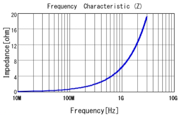
■ LQG15WH1N0B02 |Z|
