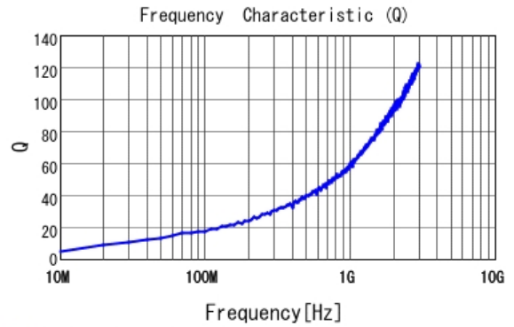
■ LQG15WH1N0B02 Q
