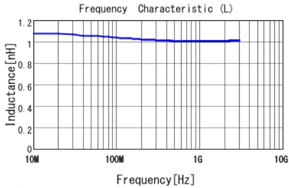
■ LQG15WH1N0B02 L
