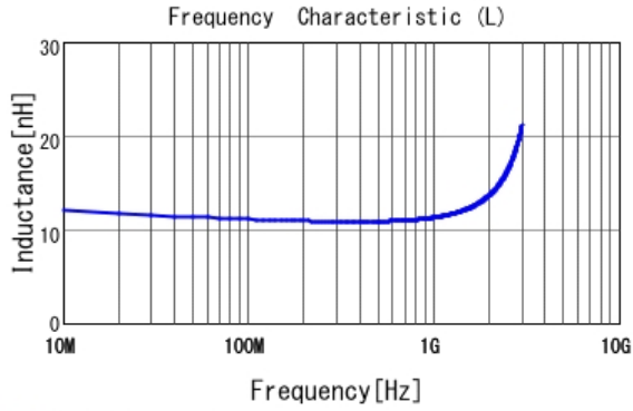
■ LQG15WH11NH02 L
