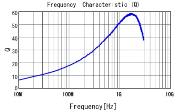
■ LQG15WH11NH02 Q
