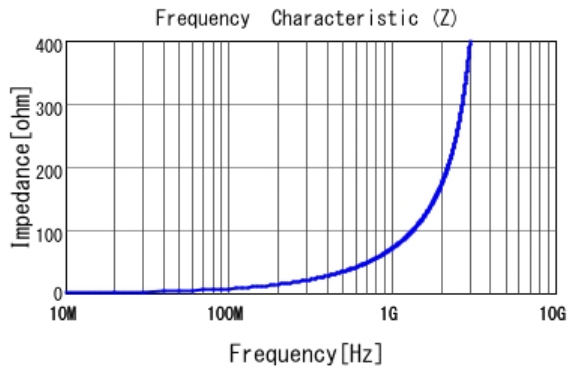
■ LQG15WH11NH02 |Z|
