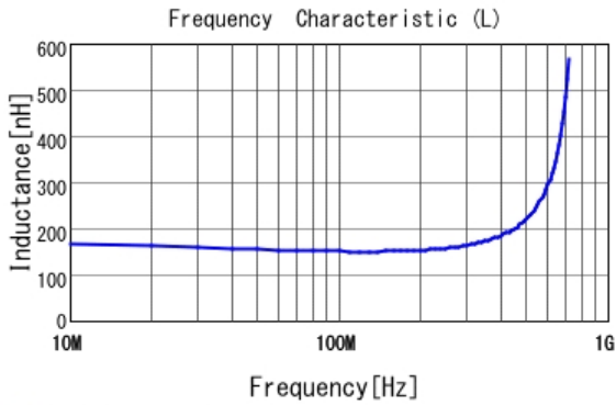
■ LQG15HZR15J02 L
