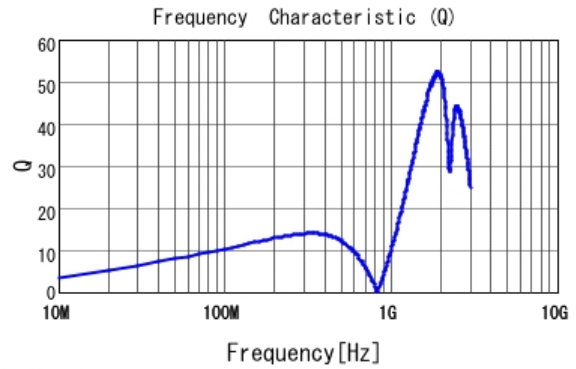
■ LQG15HZR15J02 Q
