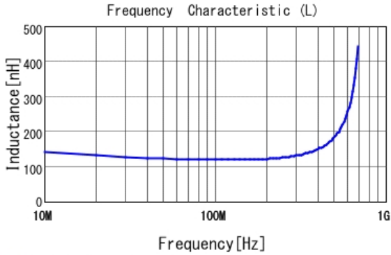
■ LQG15HZR12J02 L
