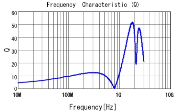
■ LQG15HZR12J02 Q
