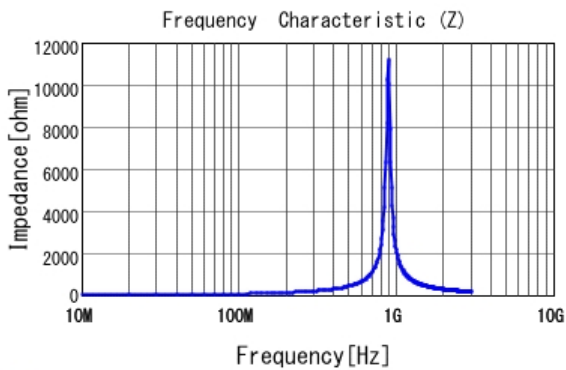
■ LQG15HZR10J02 |Z|
