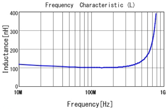
■ LQG15HZR10J02 L
