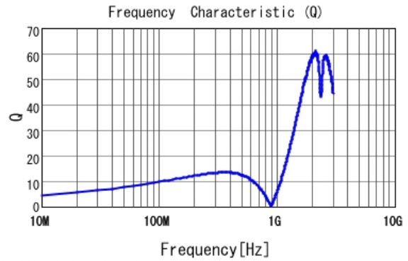
■ LQG15HZR10J02 Q
