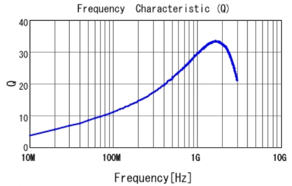
■ LQG15HZ8N2J02 Q
