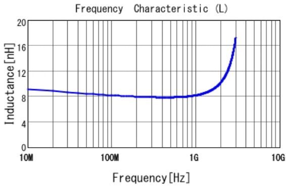
■ LQG15HZ8N2J02 L
