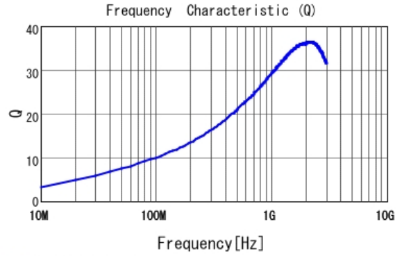
■ LQG15HZ6N2S02 Q
