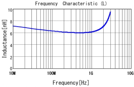
■ LQG15HZ6N2S02 L
