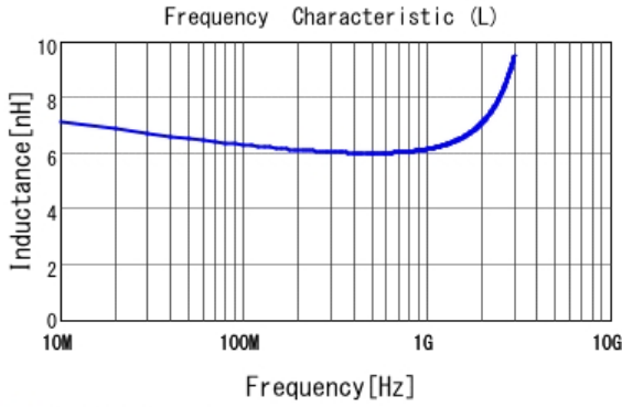
■ LQG15HZ6N2C02 L
