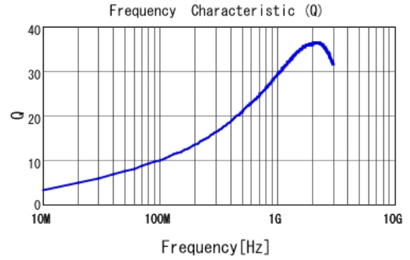
■ LQG15HZ6N2C02 Q
