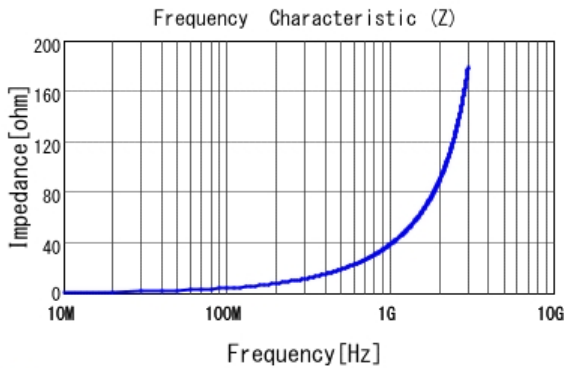
■ LQG15HZ6N2C02 |Z|
