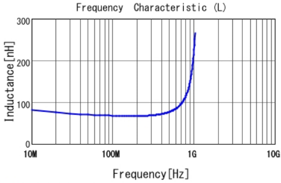
■ LQG15HZ68NJ02 L
