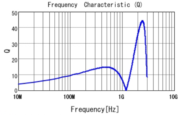
■ LQG15HZ68NJ02 Q
