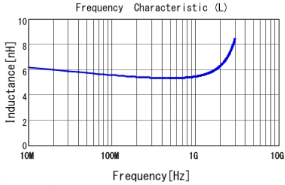
■ LQG15HZ5N6S02 L
