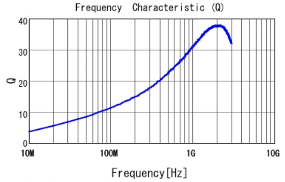
■ LQG15HZ5N6S02 Q
