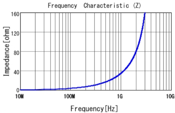
■ LQG15HZ5N6S02 |Z|
