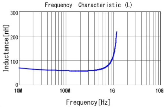
■ LQG15HZ56NJ02 L
