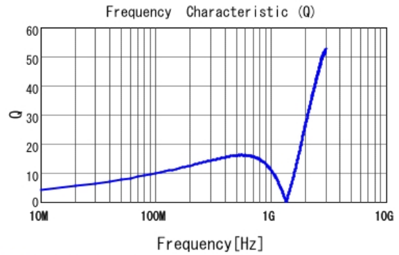
■ LQG15HZ56NJ02 Q
