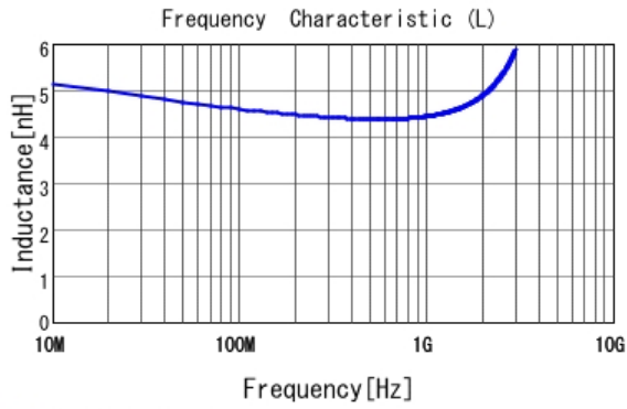
■ LQG15HZ4N7S02 L
