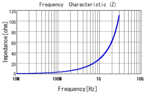
■ LQG15HZ4N7S02 |Z|
