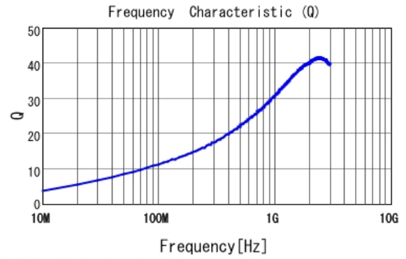
■ LQG15HZ4N7S02 Q
