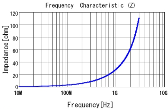
■ LQG15HZ4N7C02 |Z|
