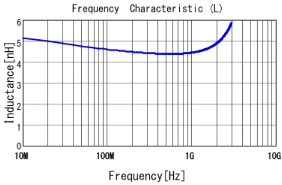
■ LQG15HZ4N7C02 L
