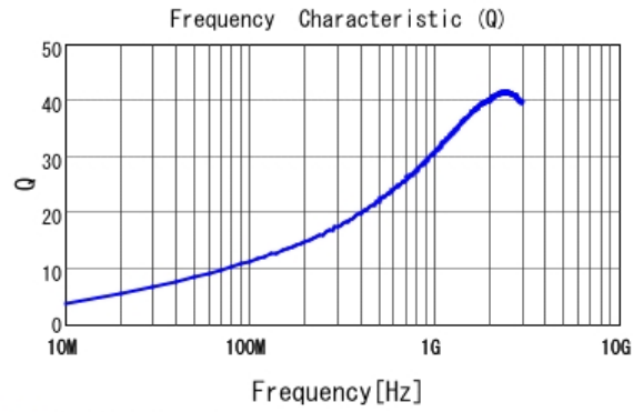
■ LQG15HZ4N7C02 Q
