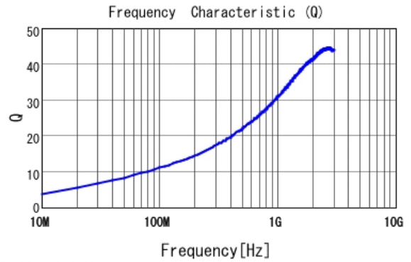
■ LQG15HZ3N9S02 Q
