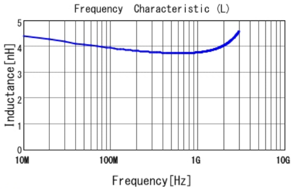
■ LQG15HZ3N9S02 L
