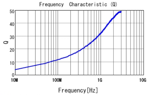
■ LQG15HZ2N7S02 Q
