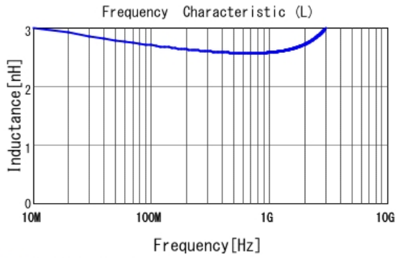
■ LQG15HZ2N7S02 L
