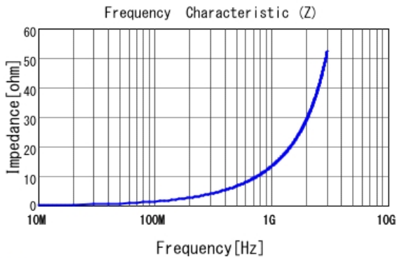
■ LQG15HZ2N2S02 |Z|
