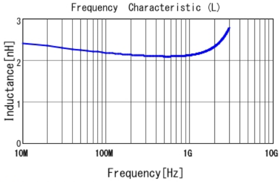
■ LQG15HZ2N2S02 L
