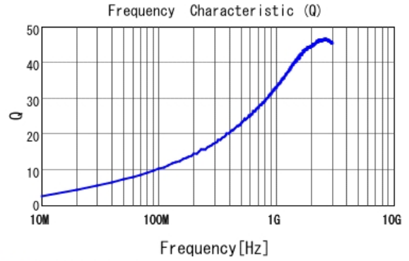
■ LQG15HZ2N2S02 Q
