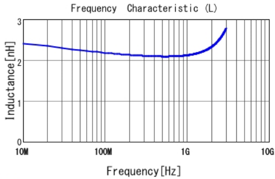
■ LQG15HZ2N2B02 L
