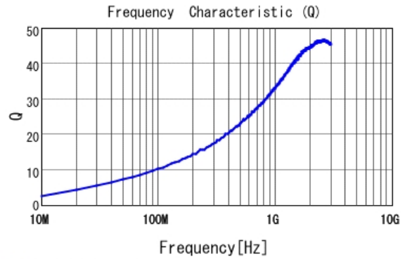
■ LQG15HZ2N2B02 Q
