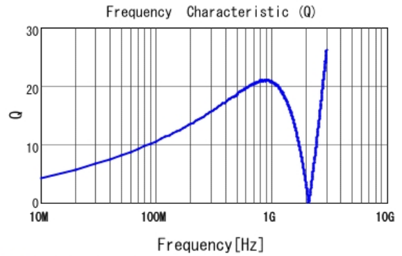
■ LQG15HZ27NJ02 Q
