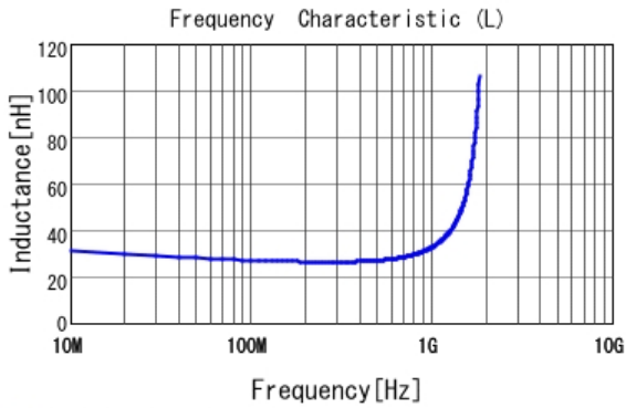
■ LQG15HZ27NJ02 L
