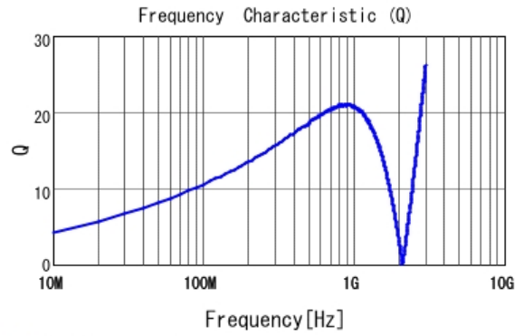
■ LQG15HZ27NH02 Q
