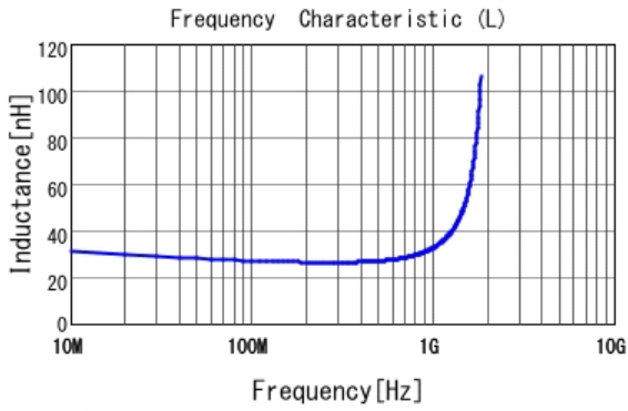
■ LQG15HZ27NH02 L
