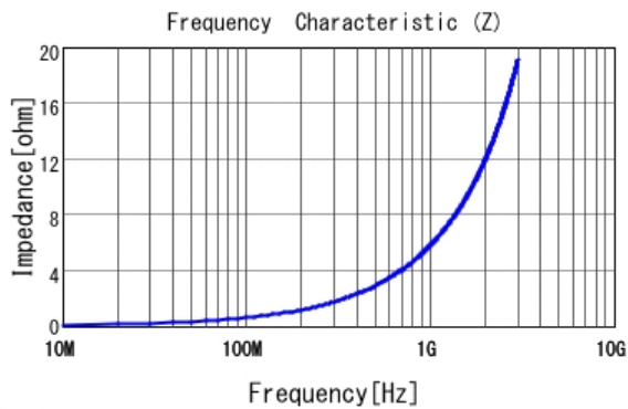
■ LQG15HZ1N0S02 |Z|
