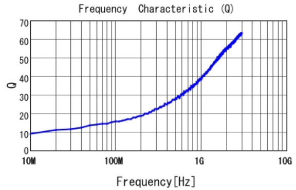
■ LQG15HZ1N0S02 Q
