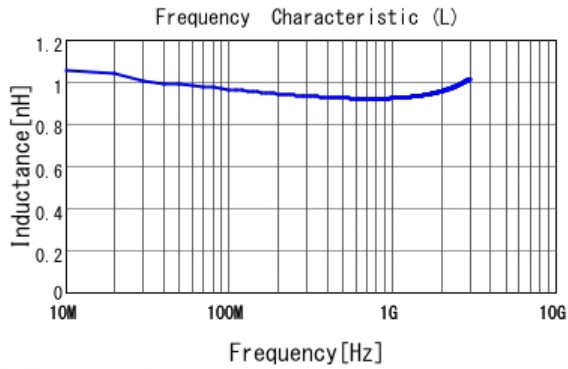
■ LQG15HZ1N0S02 L
