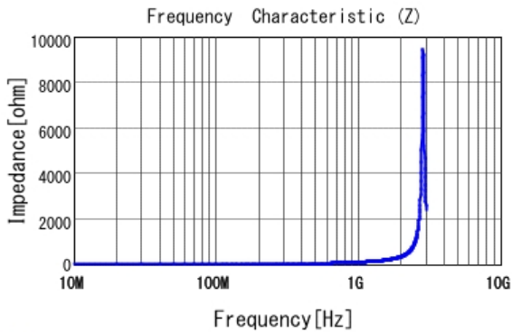
■ LQG15HZ15NJ02 |Z|
