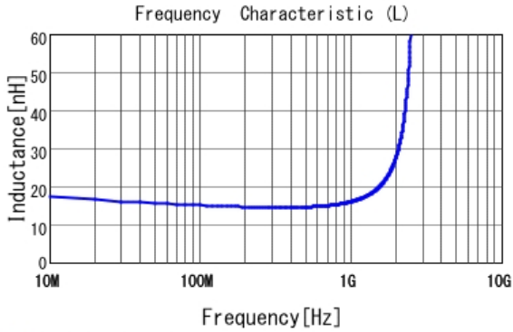
■ LQG15HZ15NJ02 L
