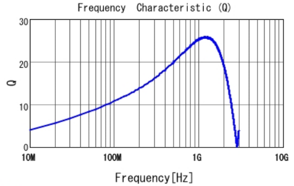
■ LQG15HZ15NJ02 Q
