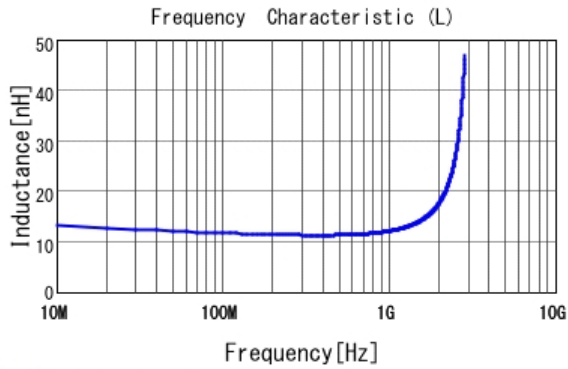
■ LQG15HZ12NJ02 L
