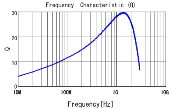
■ LQG15HZ12NJ02 Q
