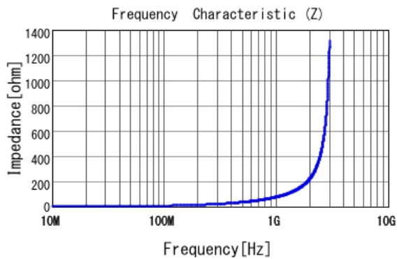
■ LQG15HZ12NJ02 |Z|
