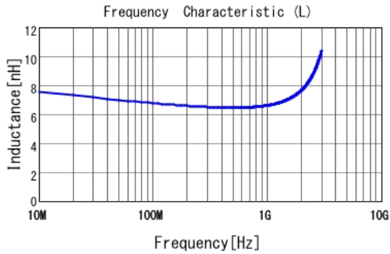
■ LQG15HS6N8H02 L
