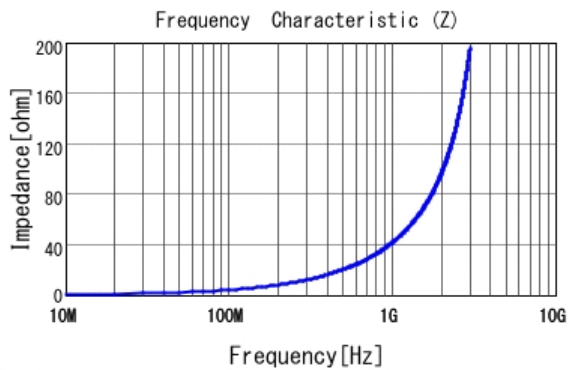
■ LQG15HS6N8H02 |Z|
