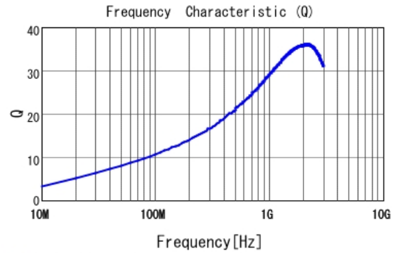
■ LQG15HS6N8H02 Q
