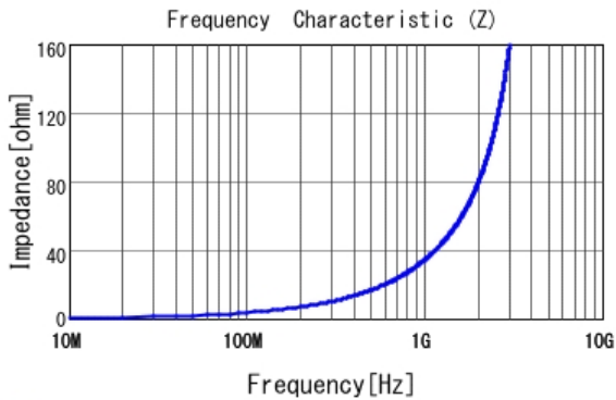
■ LQG15HS5N6C02 |Z|
