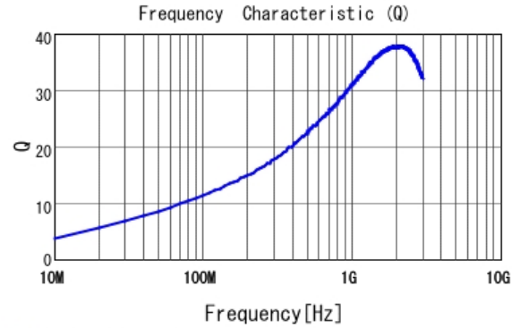
■ LQG15HS5N6C02 Q
