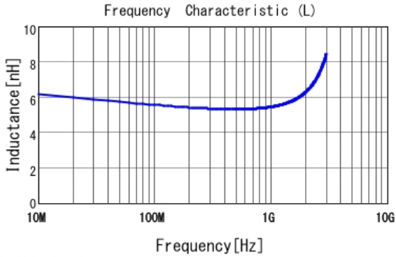
■ LQG15HS5N6C02 L
