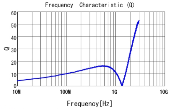
■ LQG15HS56NG02 Q
