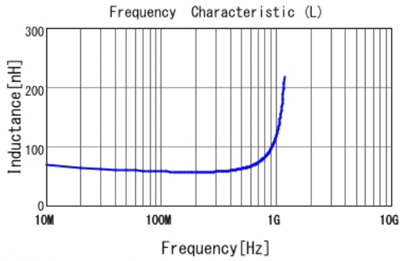
■ LQG15HS56NG02 L
