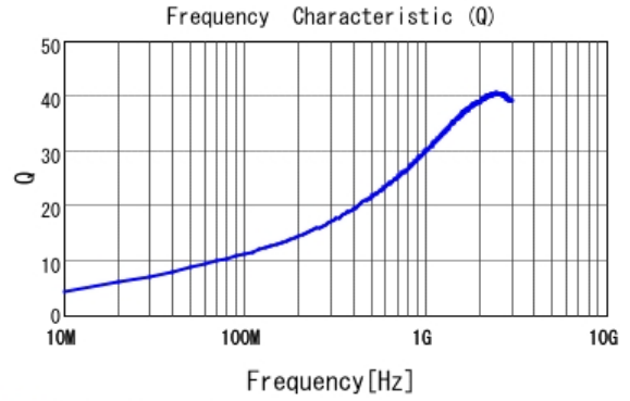
■ LQG15HS4N3B02 Q
