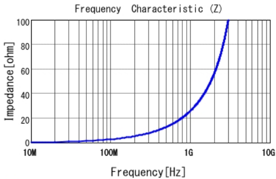
■ LQG15HS4N3B02 |Z|
