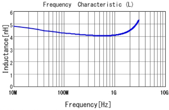
■ LQG15HS4N3B02 L
