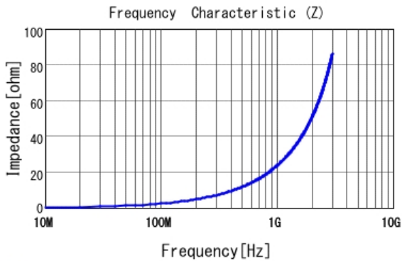
■ LQG15HS3N9C02 |Z|
