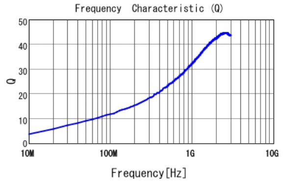
■ LQG15HS3N3C02 Q
