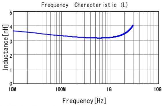
■ LQG15HS3N3C02 L
