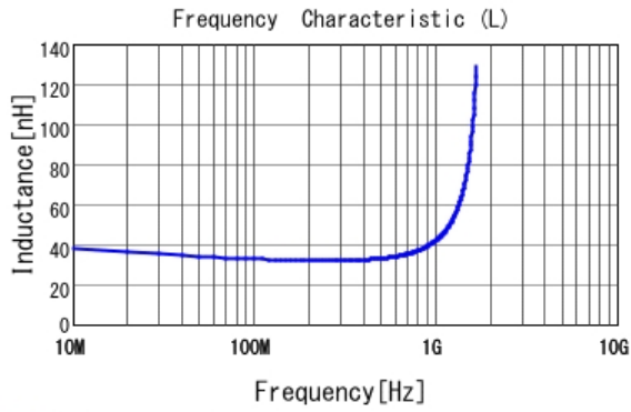
■ LQG15HS33NG02 L
