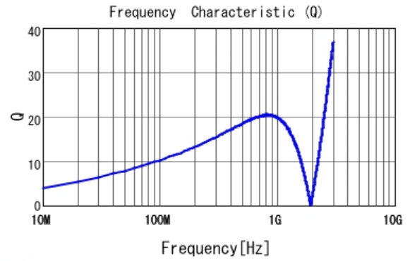
■ LQG15HS33NG02 Q
