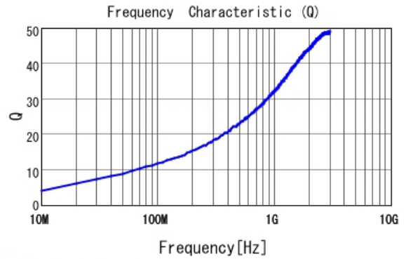
■ LQG15HS2N7C02 Q
