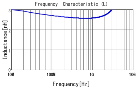
■ LQG15HS2N7C02 L
