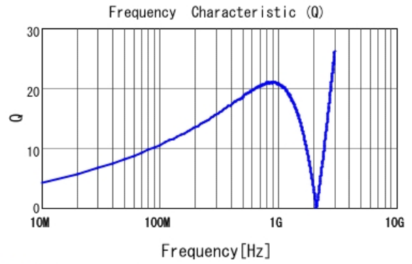
■ LQG15HS27NG02 Q
