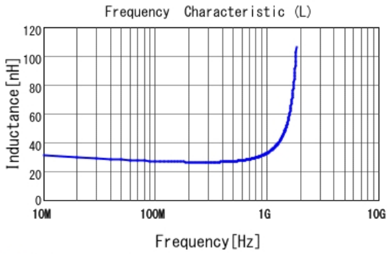
■ LQG15HS27NG02 L
