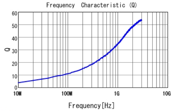
■ LQG15HS1N6B02 Q
