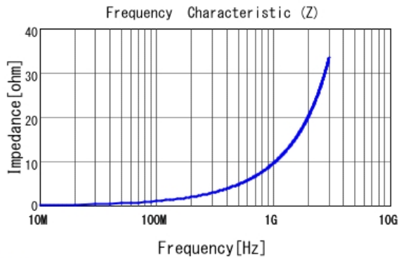
■ LQG15HS1N6B02 |Z|
