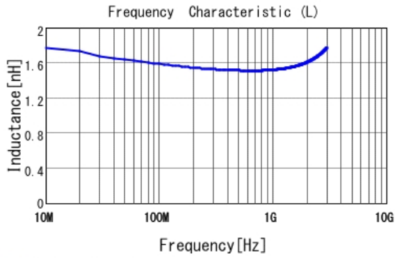
■ LQG15HS1N6B02 L
