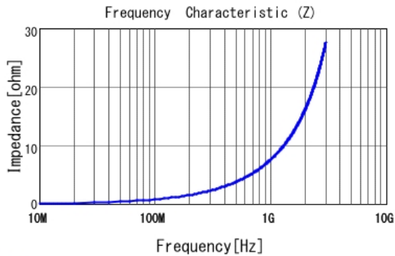
■ LQG15HS1N3B02 |Z|
