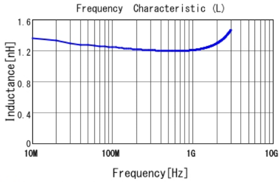
■ LQG15HS1N3B02 L
