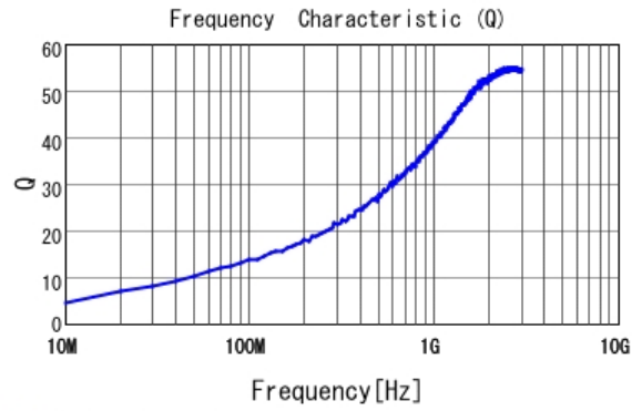
■ LQG15HS1N3B02 Q
