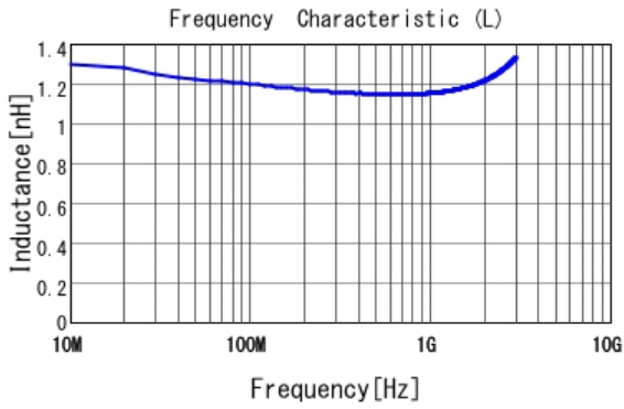
■ LQG15HS1N2C02 L
