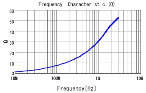
■ LQG15HS1N2C02 Q
