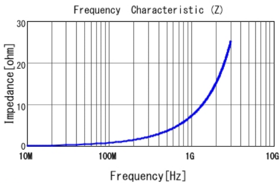
■ LQG15HS1N2C02 |Z|
