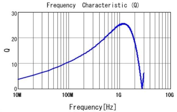
■ LQG15HS18NH02 Q
