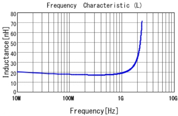
■ LQG15HS18NH02 L
