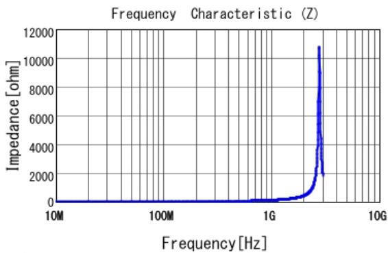
■ LQG15HS18NH02 |Z|
