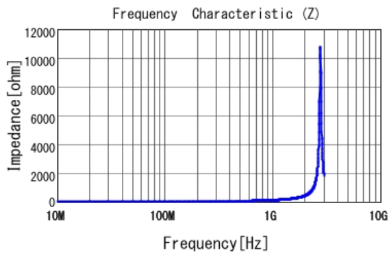
■ LQG15HS18NG02 |Z|
