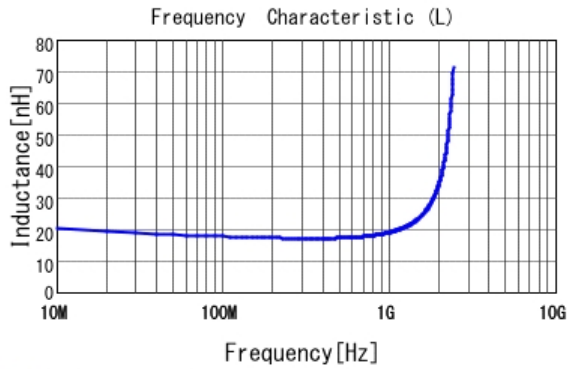
■ LQG15HS18NG02 L
