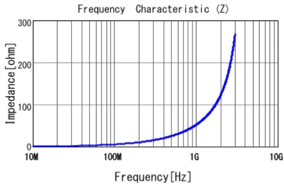
■ LQG15HN8N2H02 |Z|
