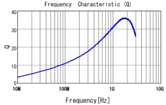
■ LQG15HN8N2H02 Q
