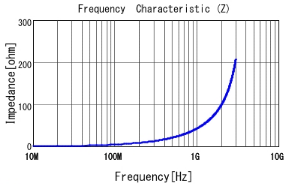
■ LQG15HN6N8H02 |Z|
