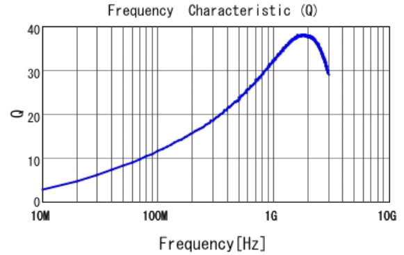
■ LQG15HN6N8H02 Q
