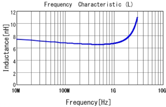
■ LQG15HN6N8H02 L
