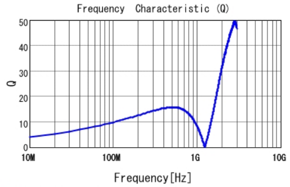
■ LQG15HN68NH02 Q
