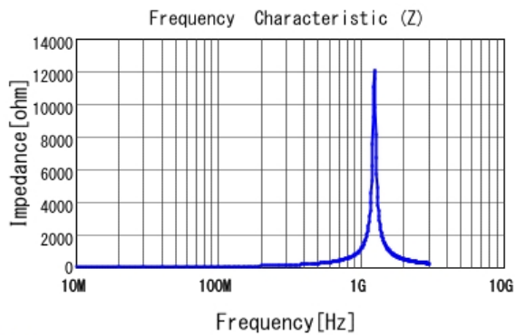
■ LQG15HN68NH02 |Z|
