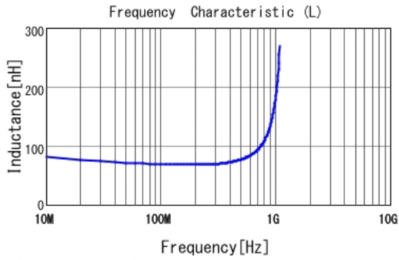
■ LQG15HN68NH02 L
