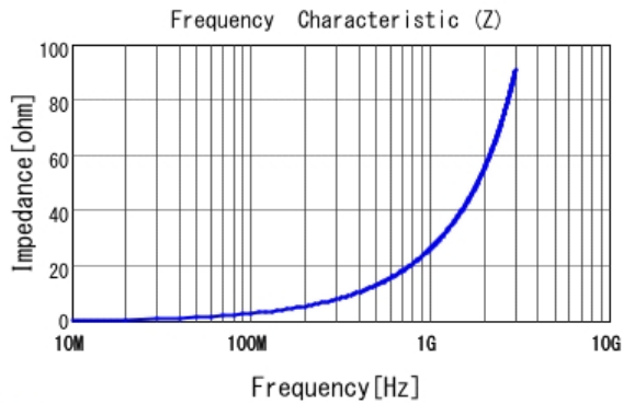
■ LQG15HN4N3B02 |Z|
