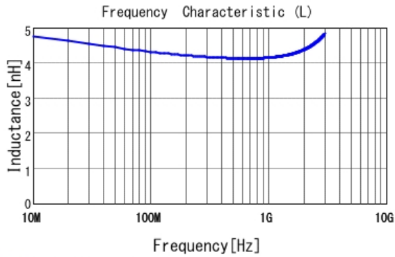
■ LQG15HN4N3B02 L
