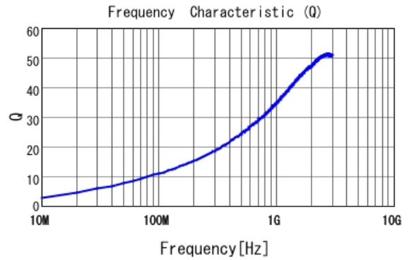
■ LQG15HN4N3B02 Q
