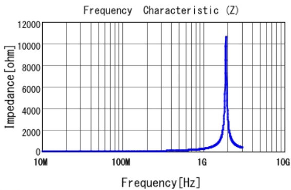
■ LQG15HN33NG02 |Z|
