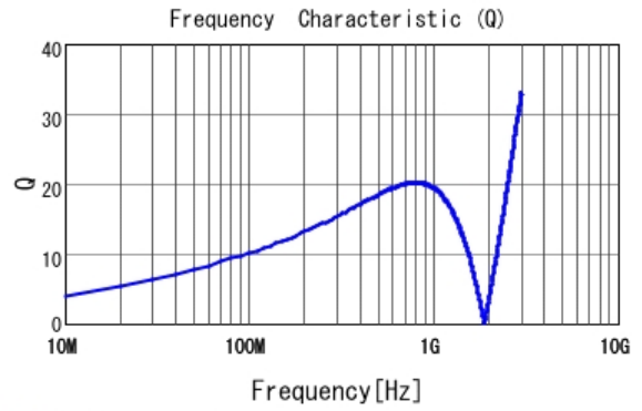
■ LQG15HN33NG02 Q
