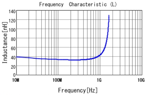
■ LQG15HN33NG02 L
