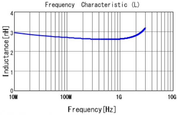
■ LQG15HN2N7S02 L
