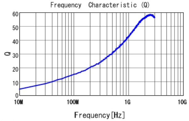
■ LQG15HN2N7S02 Q
