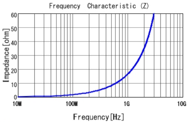
■ LQG15HN2N7S02 |Z|
