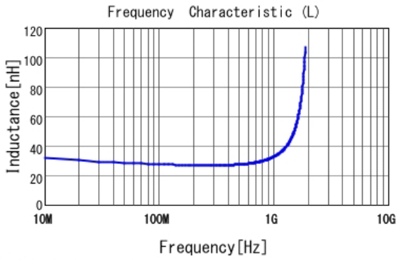
■ LQG15HN27NG02 L
