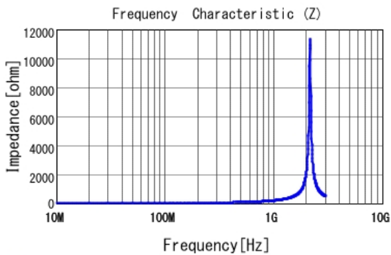
■ LQG15HN27NG02 |Z|
