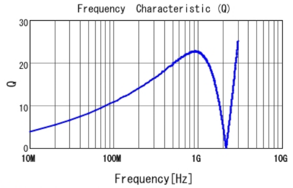
■ LQG15HN27NG02 Q
