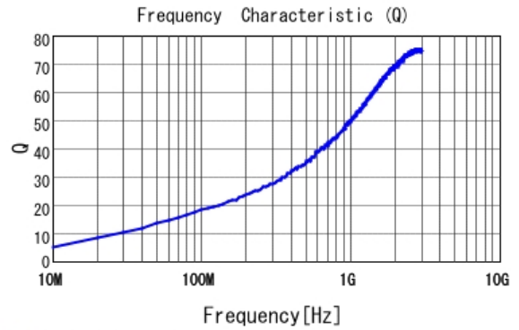
■ LQG15HN1N8C02 Q
