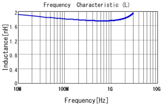
■ LQG15HN1N8C02 L
