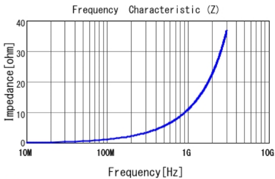
■ LQG15HN1N8C02 |Z|
