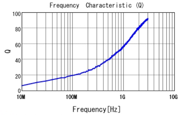
■ LQG15HN1N5B02 Q
