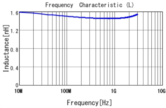
■ LQG15HN1N5B02 L
